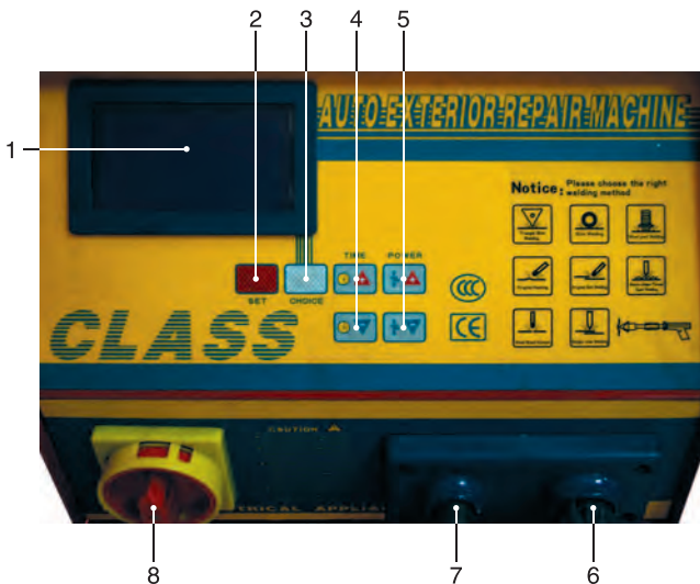
Рисунок 3 – Панель управления
